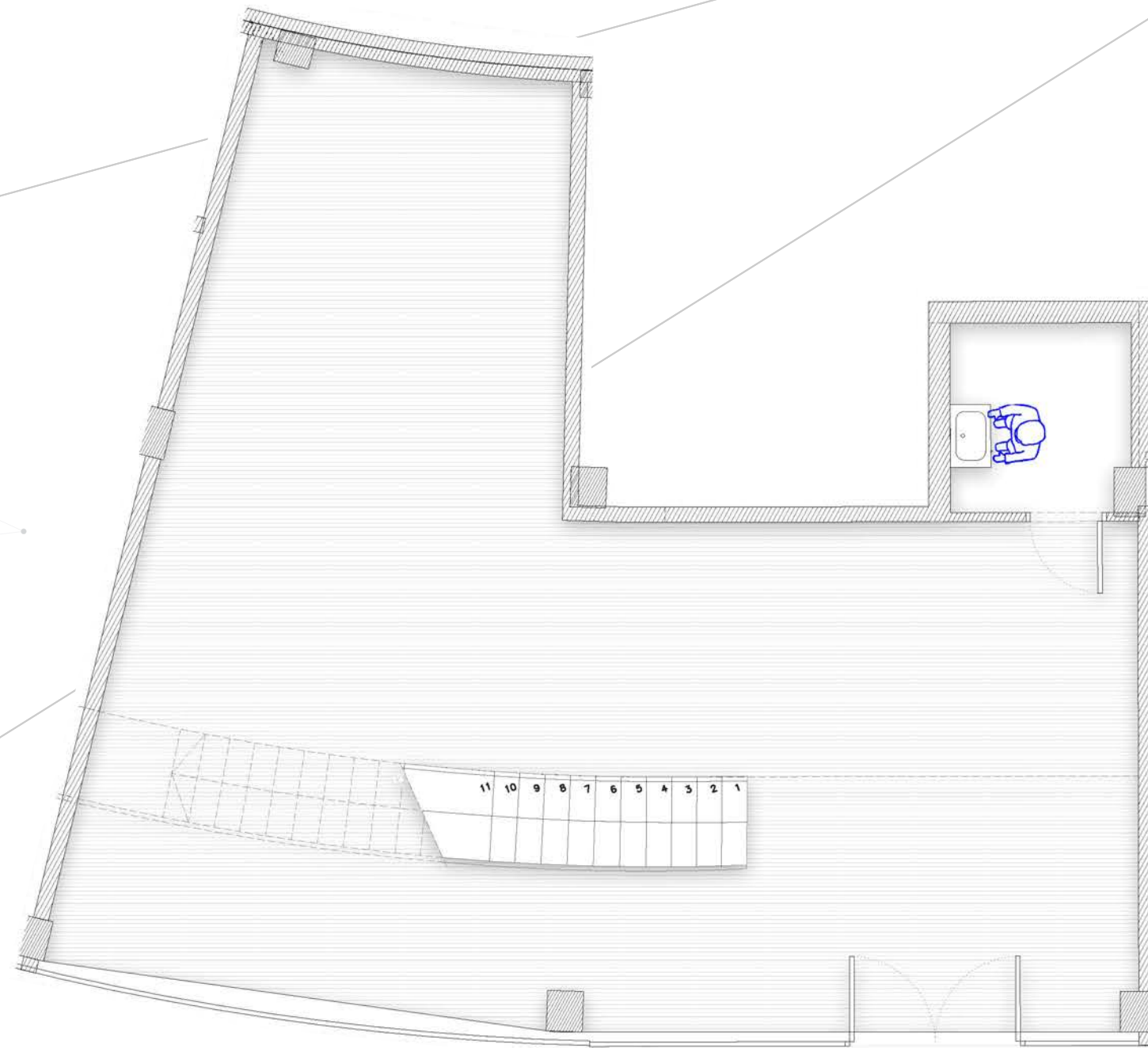
Planta Baixa
